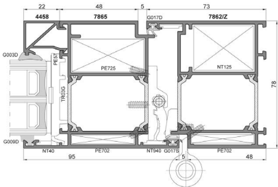
Przekrój drzwi Procural PE78N
